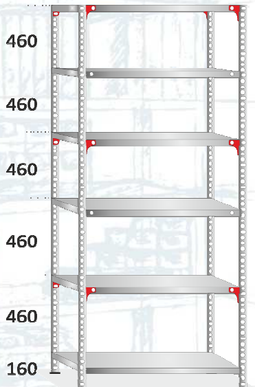
2 500 mm magas 6 polcos állvány
